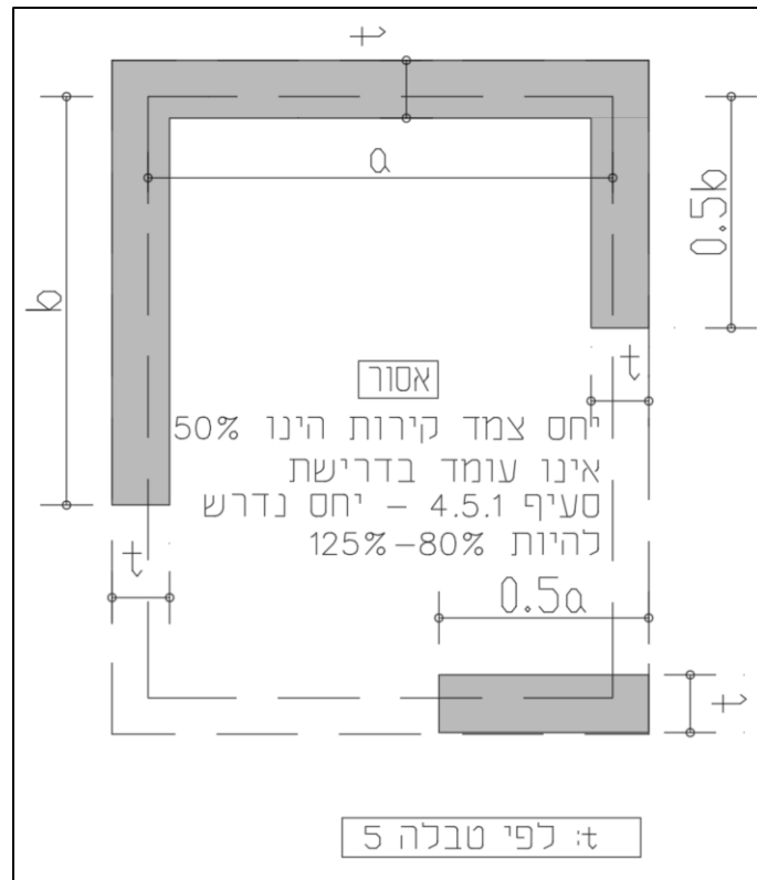
איור 31 - דוגמאות לתכנון אשר אינו עומד בתנאים עבור "מקרה מס' 1" (50%-70% היקף ירידת קירות)
