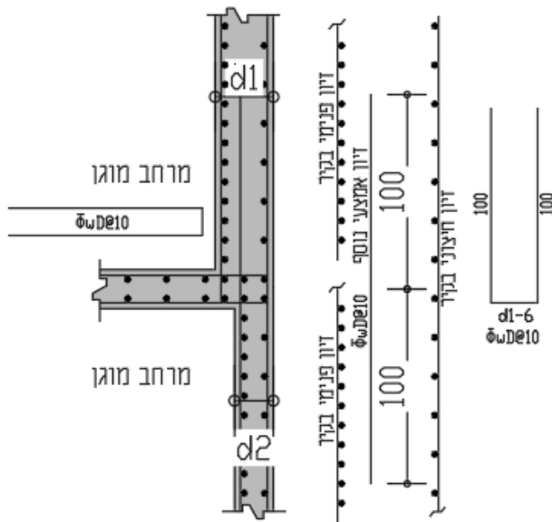
סטייה חיצונית
