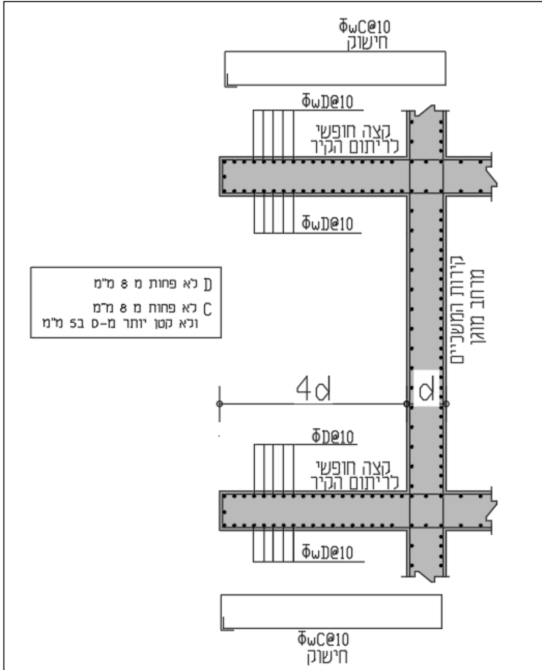
איור 5 - חתך אנכי המתאר ריתום של קיר לתקרה/רצפה או תכנית המתארת ריתום של קיר לקיר
