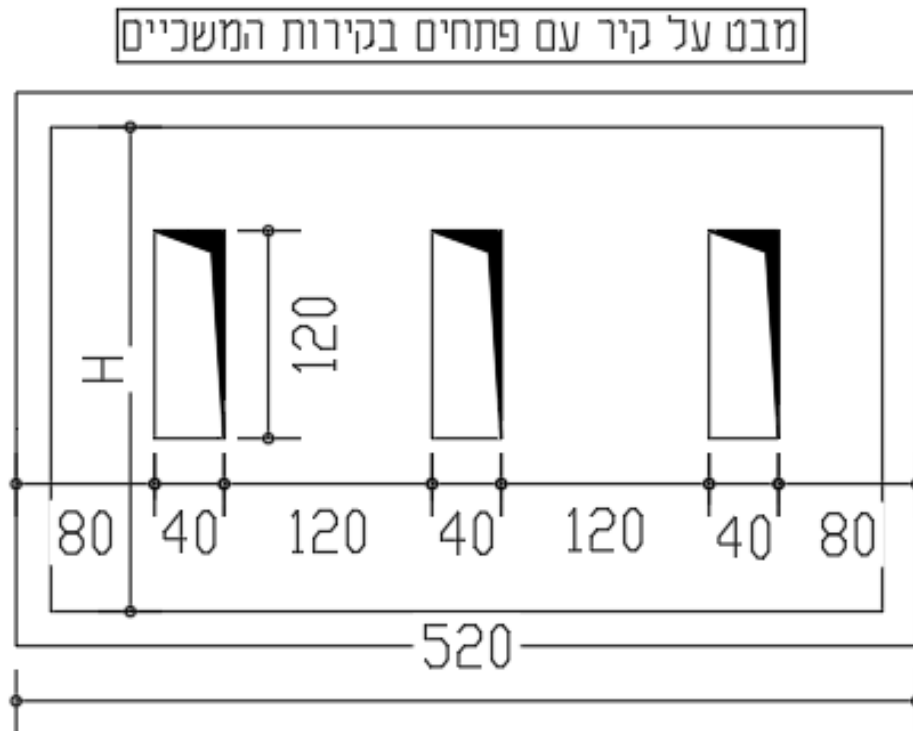
איור 13 - דוגמה לפתחים ביחס גודל שאינו תואם לדרישה ונדרש לקזז מחישוב היקף קירות
