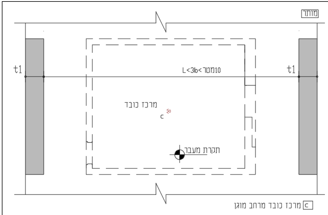
איור 38 - דוגמאות לתכנון נכון ועמידה בתנאים עבור "מקרה מס' 3" (0%-25% היקף ירידת קירות)
