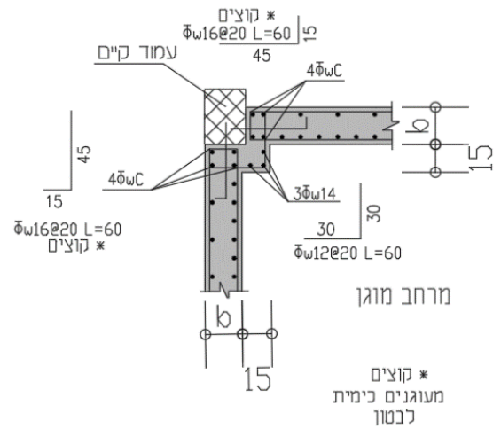
פרט עיבוי עמוד קיים
