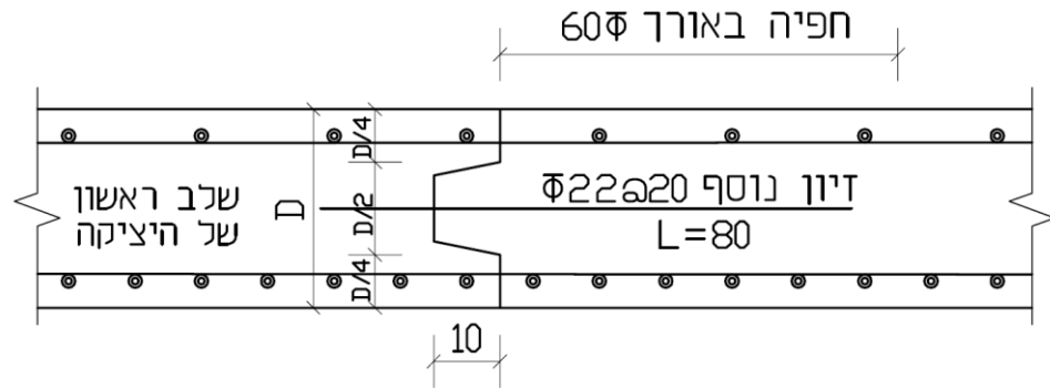
איור 43 - פרט מישק יציקה (תפר עבודה)
