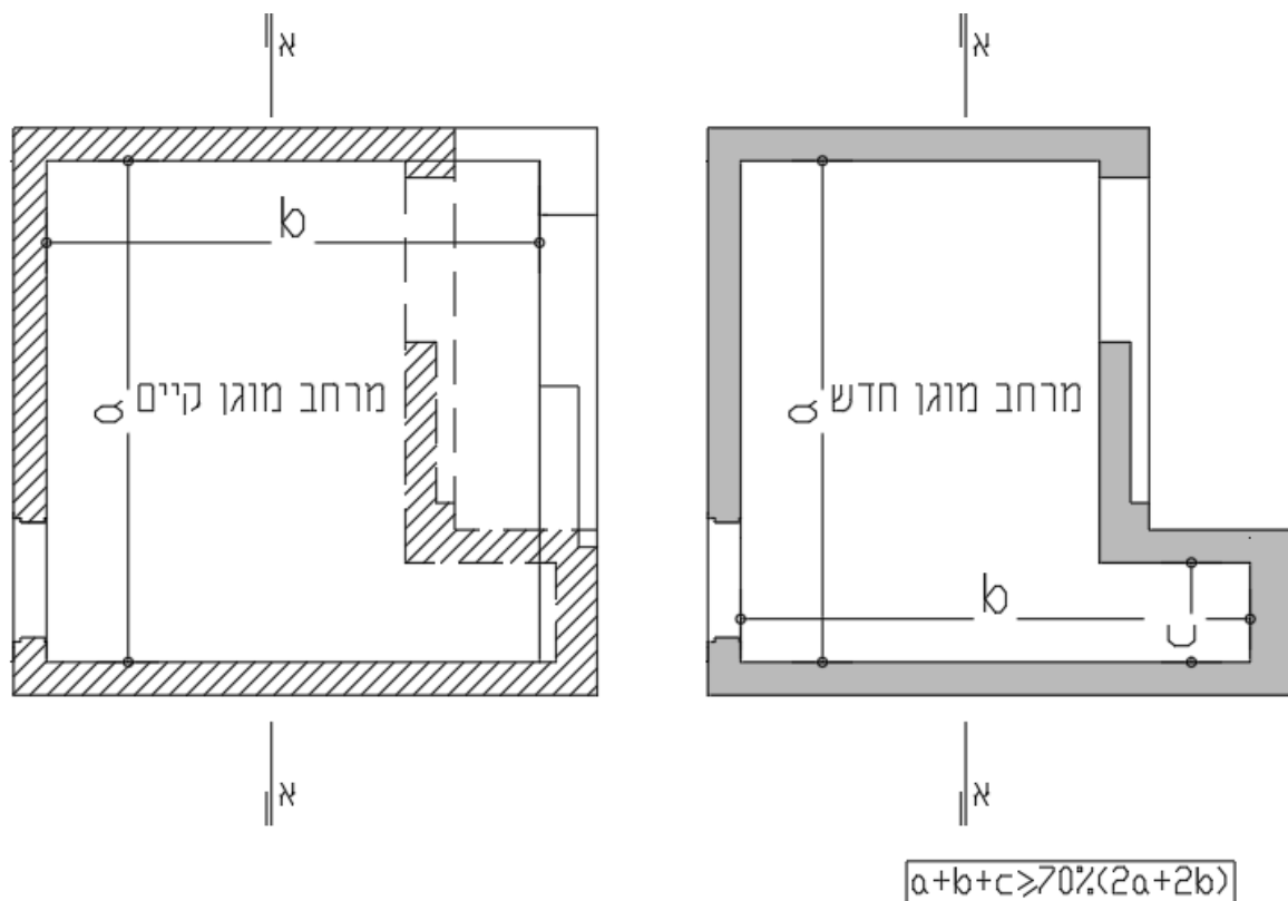
איור 46 - ירידת קירות מרחב מוגן חדש על מרחב מוגן קיים
