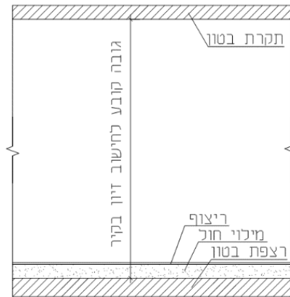
איור 6 - קביעת גובה קיר מרחב מוגן
