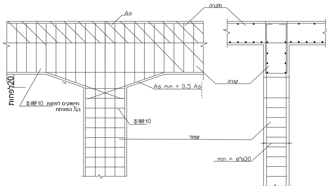
איור 50 - פרט ריתום עמוד לקורה של תקרת המרחב המוגן
