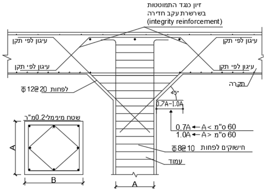
איור 49 - פרט ריתום עמוד לתקרה בתוך מרחב מוגן
