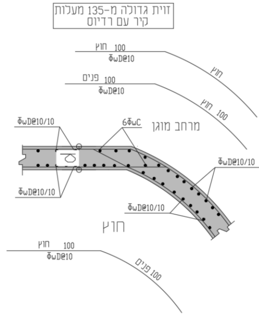
זווית קטנה מ-90 מעלות
