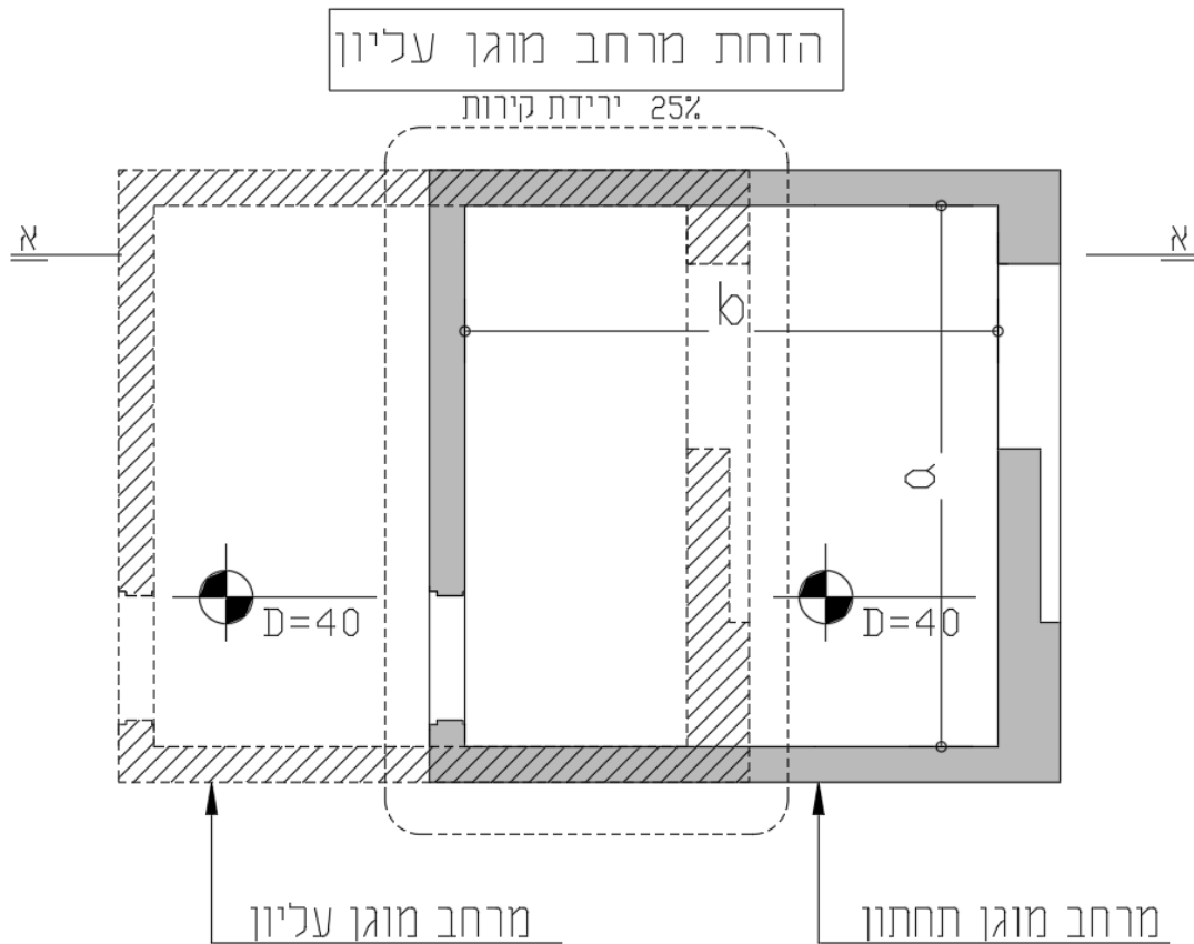
איור 21 - תוכנית - הזחה מותרת של המרחב המוגן העליון
