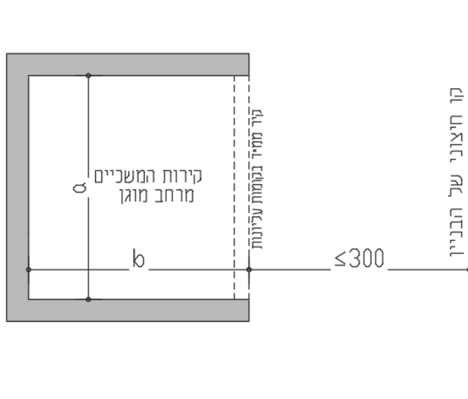
איור 15 – קירות המשך עם זיון 10/10 משני צידי הקירות
